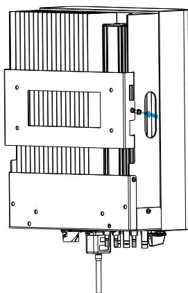
Rys. 4.6 Instalacja Inwertera
