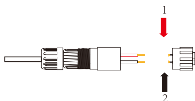
Rys. 7.5 Terminal wodoodporny
