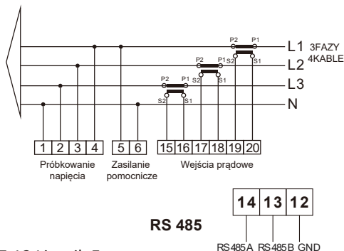
Rys. 7.13 Licznik Eastron
