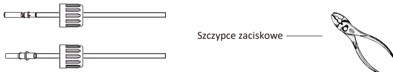
Rys. 5.4 Zaciśnij pin kontaktowe do przewodu
