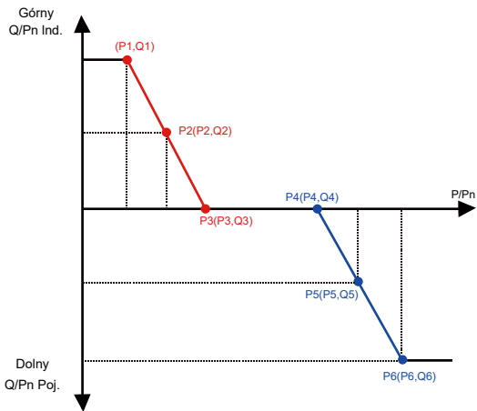
Rys. 8.39 Krzywa regulacji mocy biernej w trybie Q(P)
