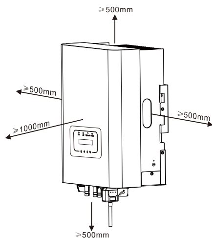
Rys. 4.3 Przerwa Instalacyjna
