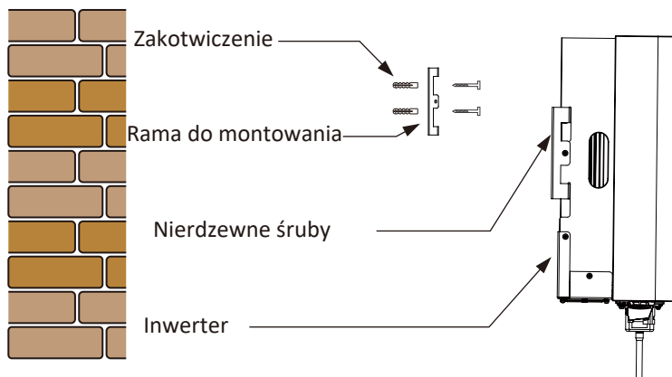
Rys. 4.4 Instalacja Inwertera
