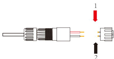
Rys. 7.5 Terminal wodoodporny
