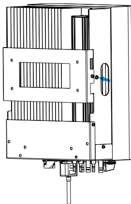
Rys. 4.6 Instalacja Inwertera
