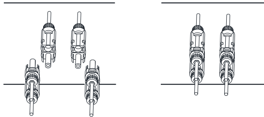
Rys. 5.6 Połączenie wejścia DC
