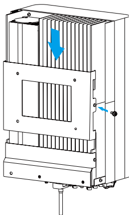
Rys. 4.6 Instalacja Inwertera
