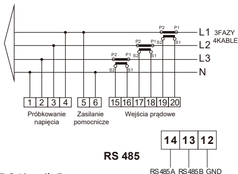
Rys. 7.3 Licznik Eastron
