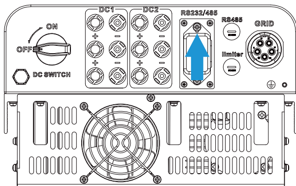
Rys. 5.13 Schemat instalacyjny rejestratora danych
