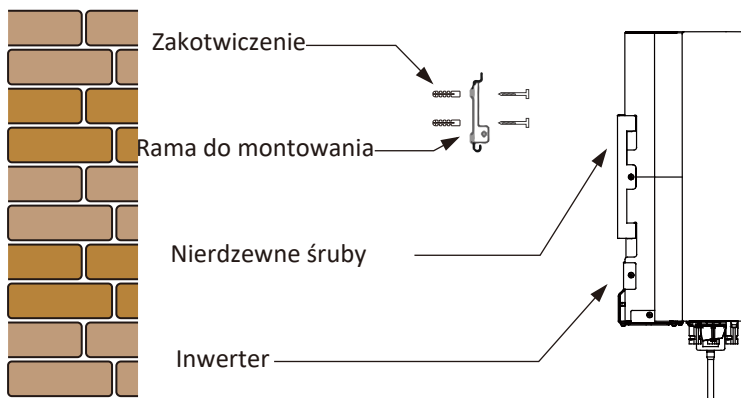
Rys. 4.4 Instalacja Inwertera
