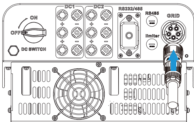
Rys. 5.10 Połączenie wejścia AC
